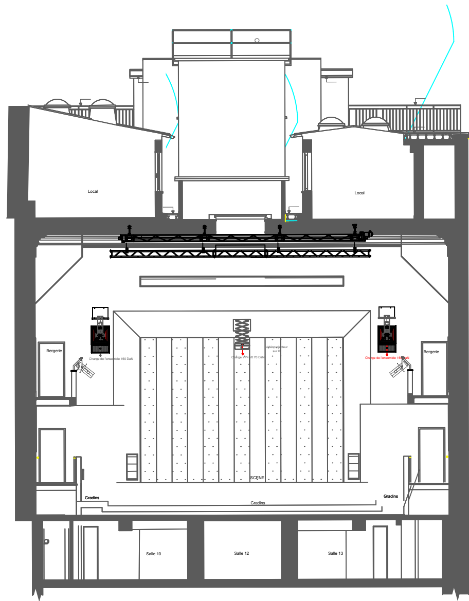
Coupe
